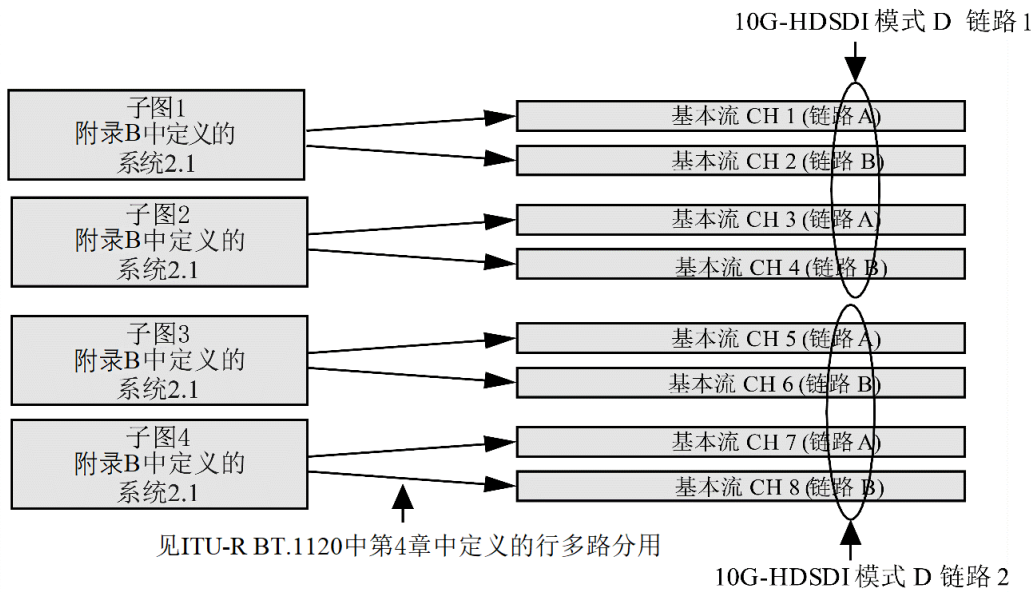
图2 系统 U1.6 的 8 路分割
