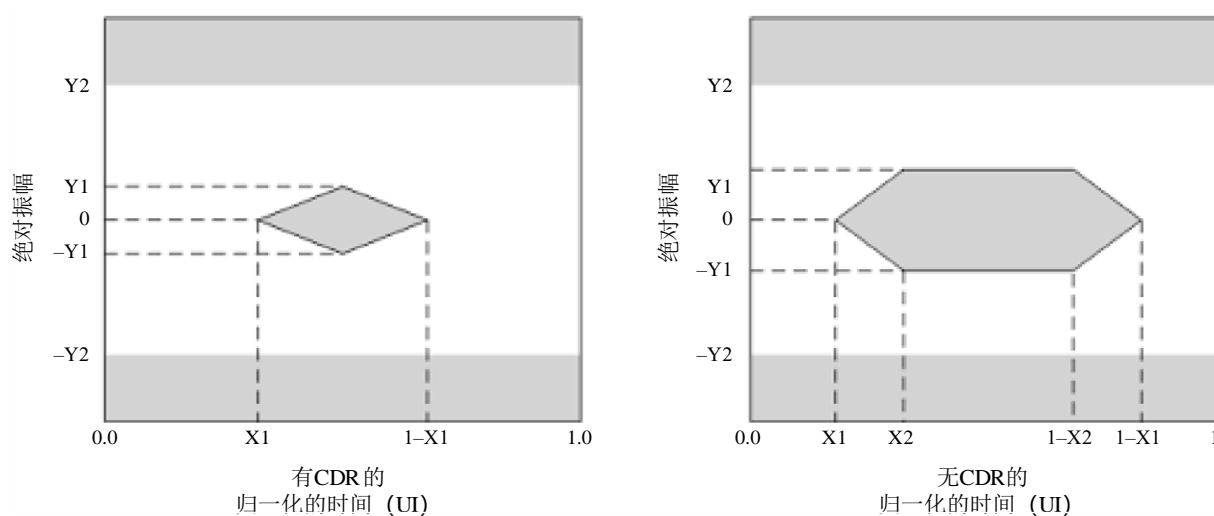
图 D.2 发射器差分输入电信号眼图
