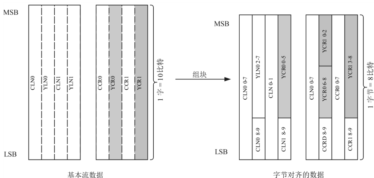
图 C.3 CRC 和 LN 字的组块
