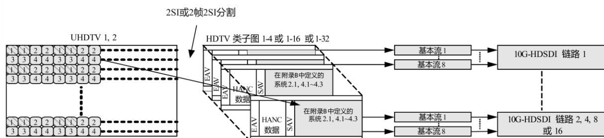
图1 UHDTV 映射概述
