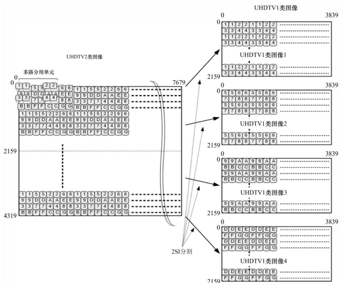
图8 UHDTV2 图像的 2SI 分割为 UHDTV1 图像
