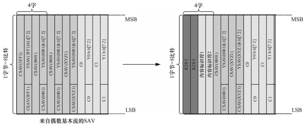
图 C.4 CH2 SAV 部分的数据替换
