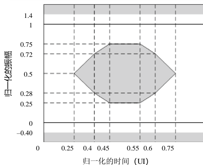
图 D.1 发射器输出光信号眼图
